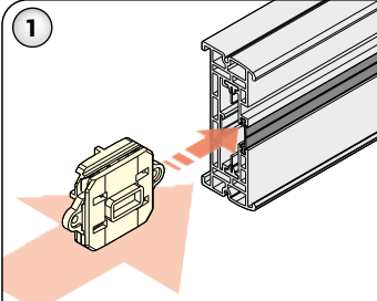
1- Ek Elemanını, iletkenler kontak arasına girecek şekilde FL-I Busbar gövdesine yerleştiriniz ve tam oturduğundan emin olunuz.
