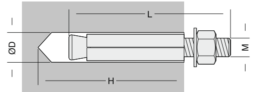
Gömlekli Dübel
